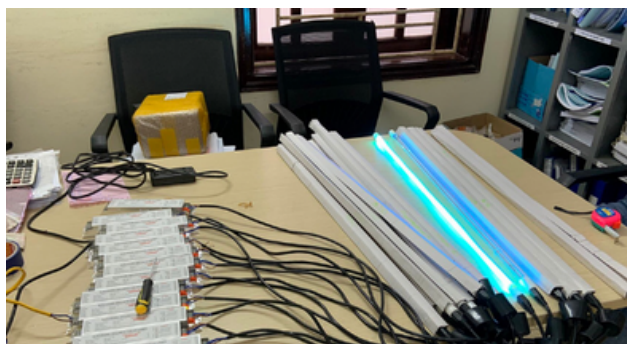
LẮP ĐẶT VÀ HOÀN THIẾT HỆ THỐNG UV XỬ LÝ NƯỚC THẢI CTY CÔNG NGHỆ XANH
